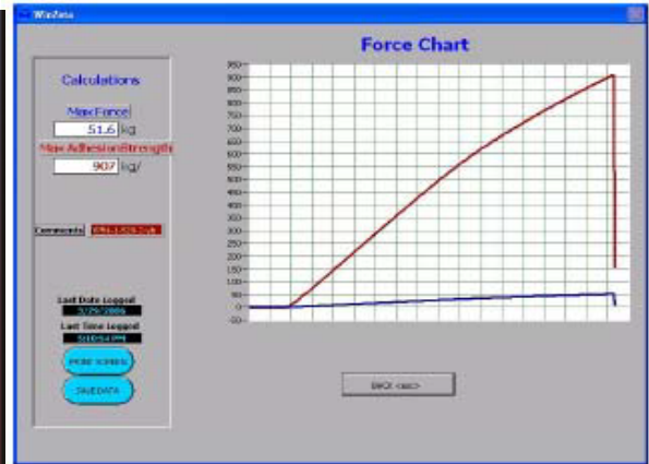
[2.7mm스타드핀을 이용한 박막밀착강도 측정에]
